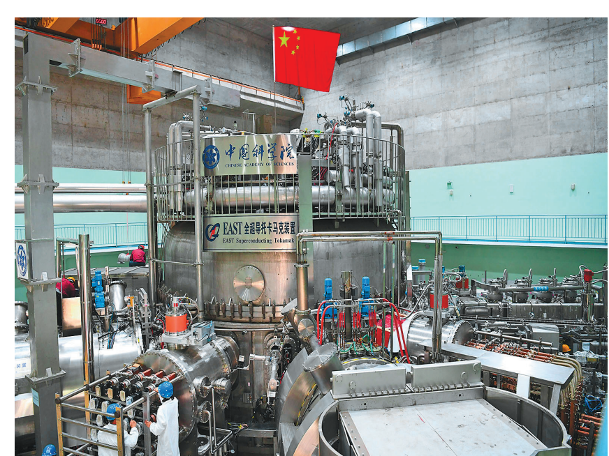
在中科院合肥物质科学研究院,工作人员对有人造太阳之称的全超导托卡马克核聚变实验装置(EAST)进行升级改造。
