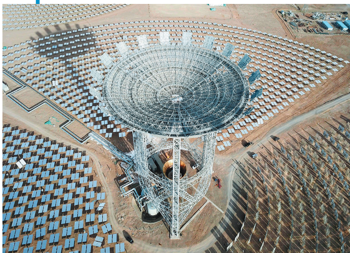
这是2021年12月8日拍摄的甘肃玉门鑫能50兆瓦熔盐塔式光热电站(无人机照片)。
