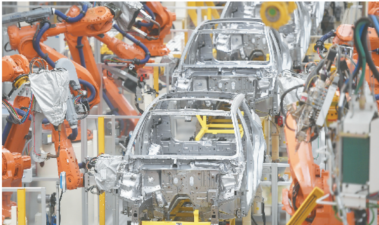
这是浙江宁波市吉利汽车春晚制造基地的自动化焊接线(2018年10月25日摄)。
